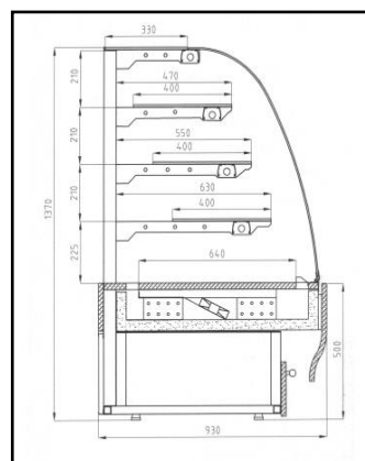
CARMELLO CGn - verze "EKO KŮŽE"
