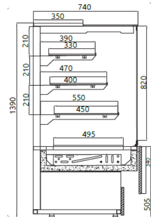
MALAGA C-PN-w - verze "MDF"
